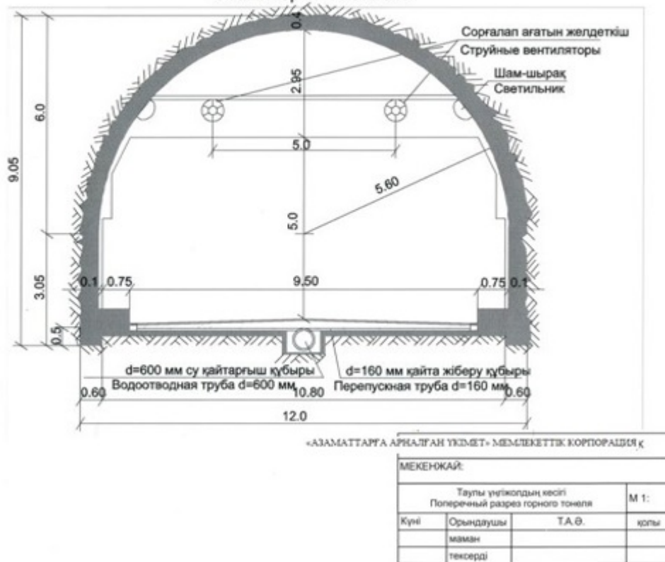
Таулы үңгірдің сұлбасы Схема горного тоннеля
