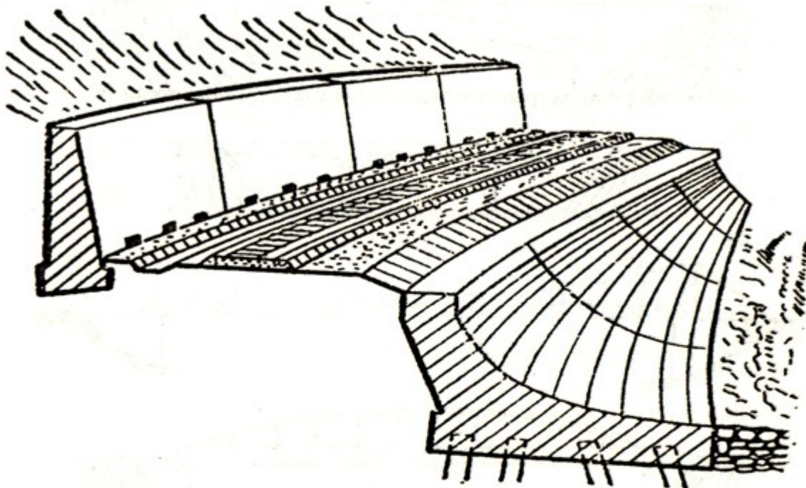
Рис. 15. Подпорные стены
