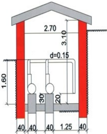
Көлденең кесік Поперечный разрез
