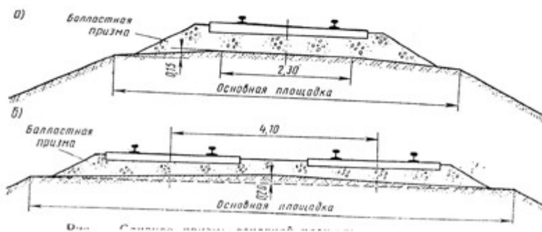
Сливная призма основной площадки земляного полотна: а – на обнопутных участках; б – на двухпутных участках
