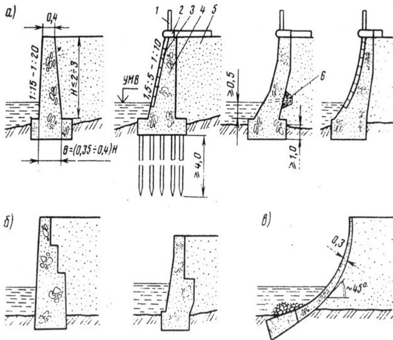
Рис.3 Поперечные сечения массивных подпорных стен городских набережных.
