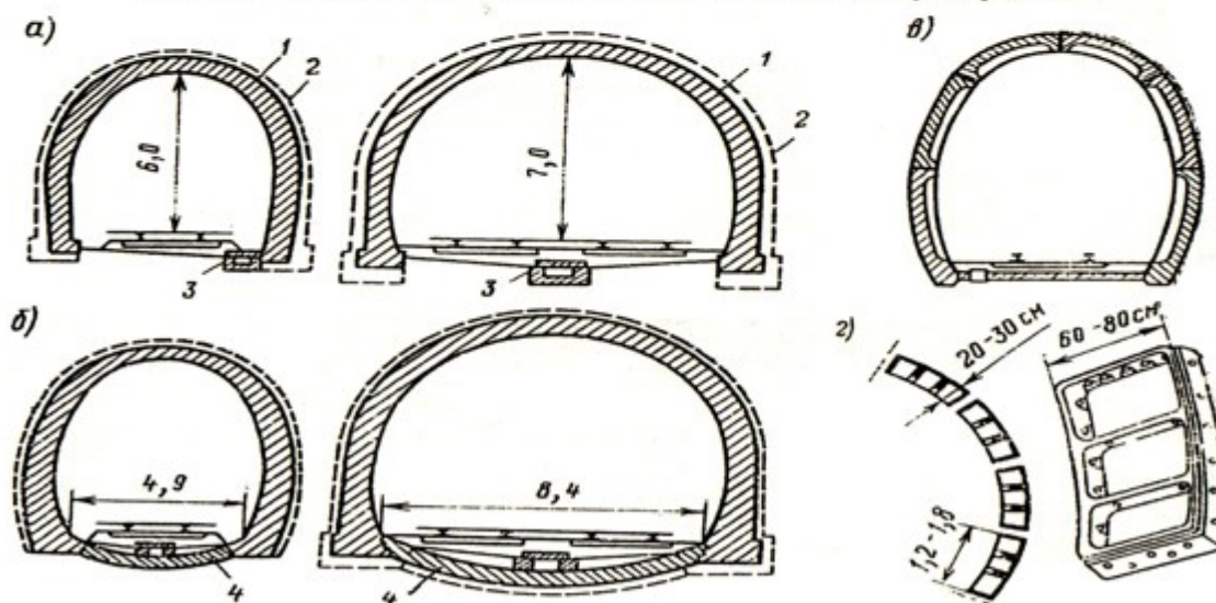
Рис. 26. Тоннельная обделка:
