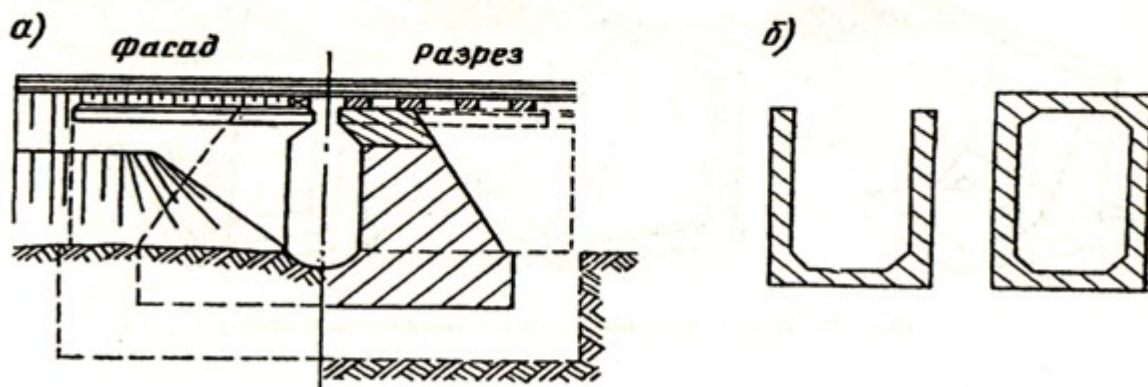
Рис. 28. Лотки:
