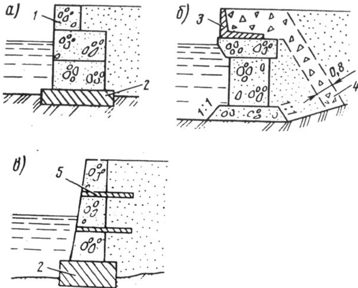
Рис.3 Сборные железобетонные подпорные стены из массивных блоков:
