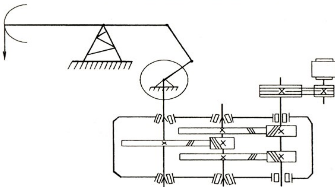
Кинематическая схема станка-качалки
