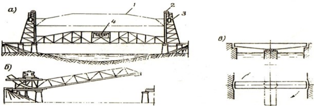
Рис. 4. Разводные мосты:
