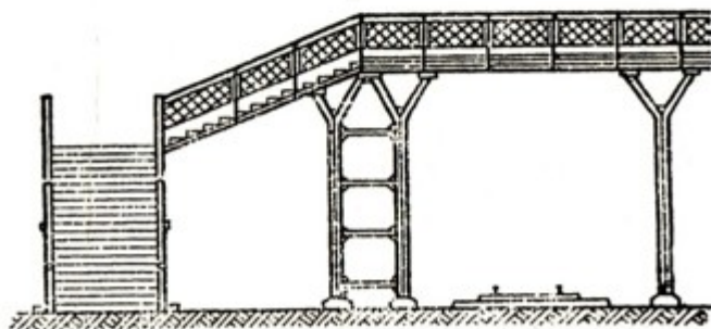
Рис. 3. Пешеходный мост
