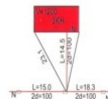
Камераның люкке байлаған сұлбасы/ Схема привязки люка камеры
