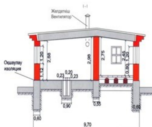
Көлденең кесік Поперечный разрез
