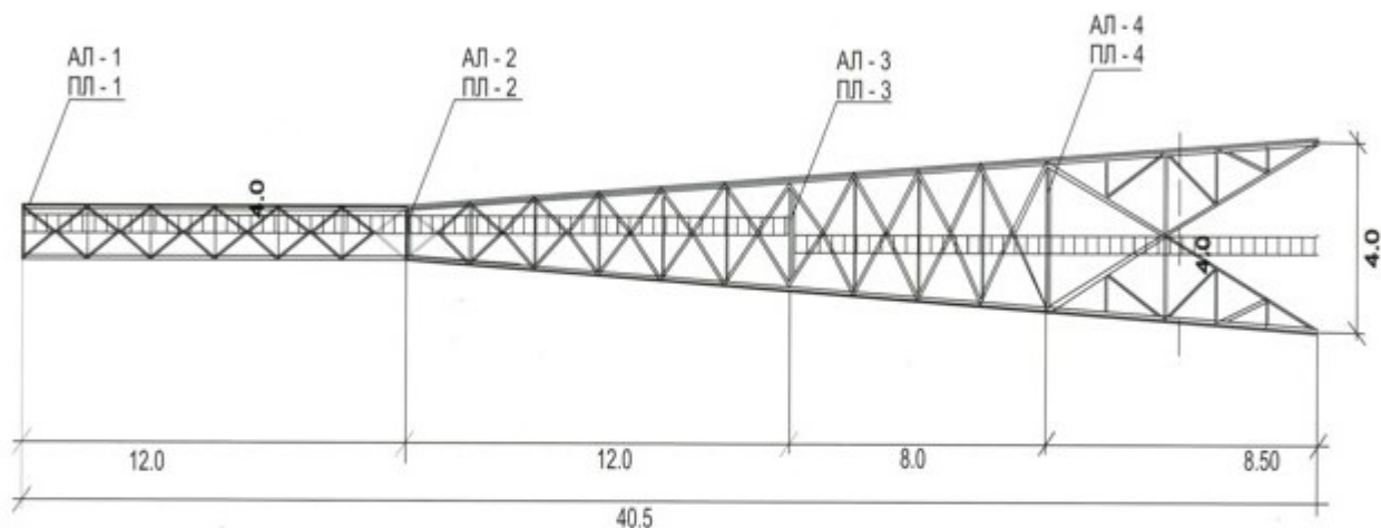
Ұялы дiңгектiң және радиорелелiк байланыстардың сұлбалық жоспары Схематический план мачты сотовой и радиорелейной связи
